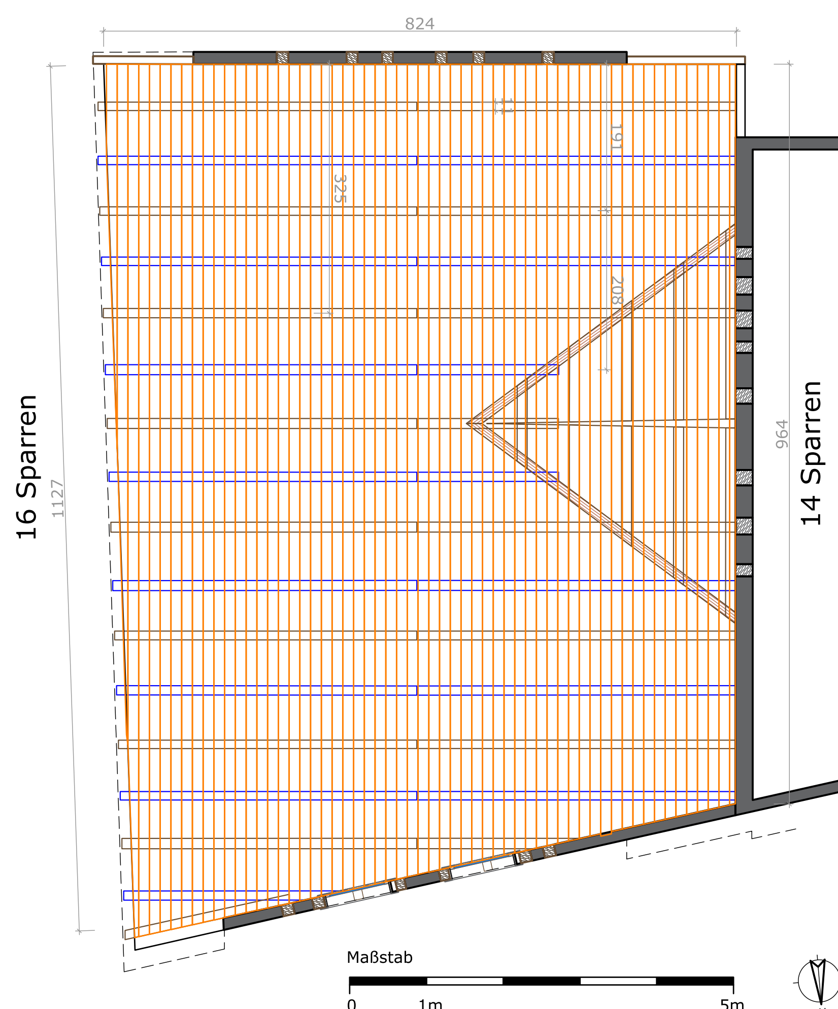
Dachstuhl Sparrenlage, Verbretteung mit Bohlen
