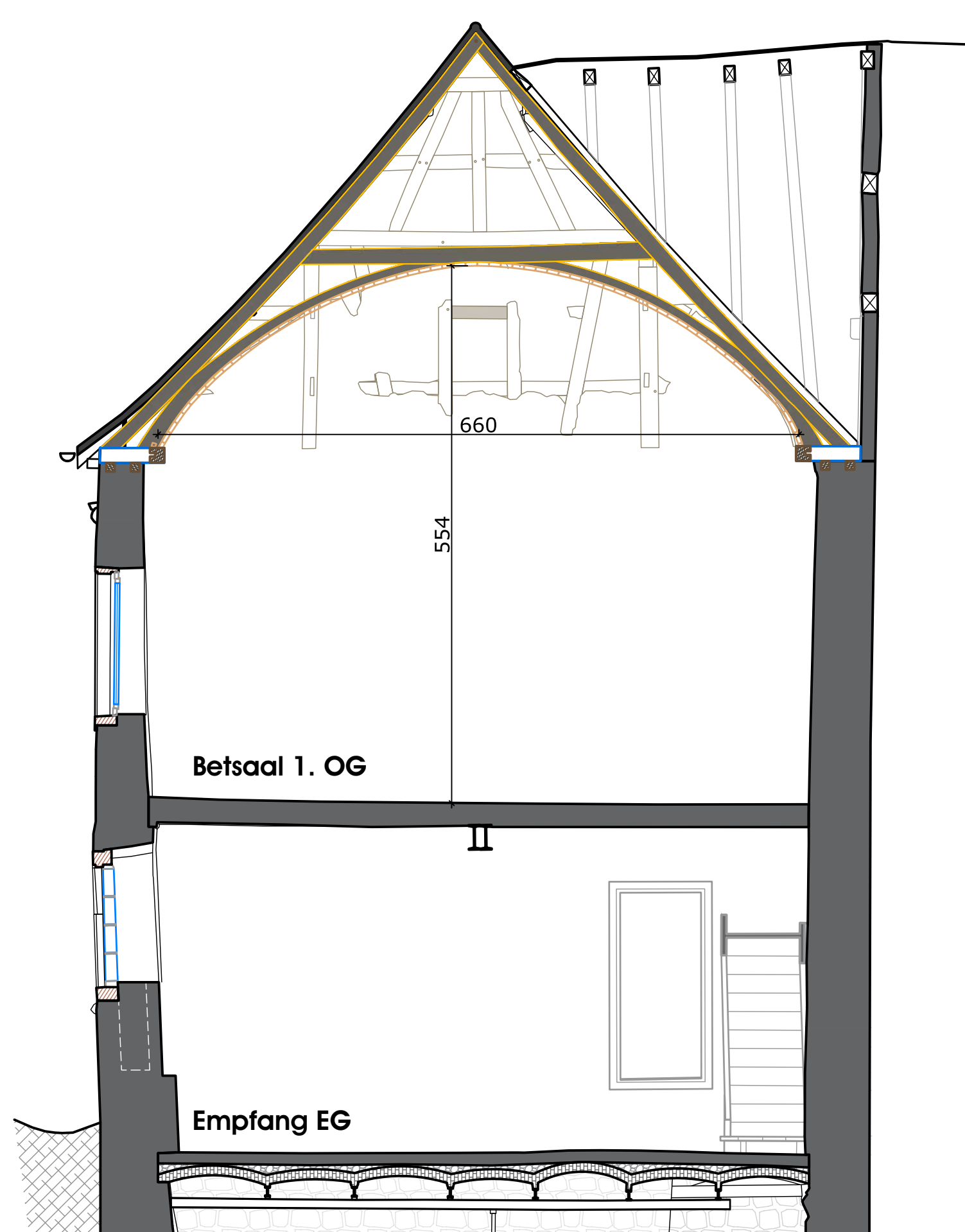
Dimension des Betsaal, Ansicht Südwand
